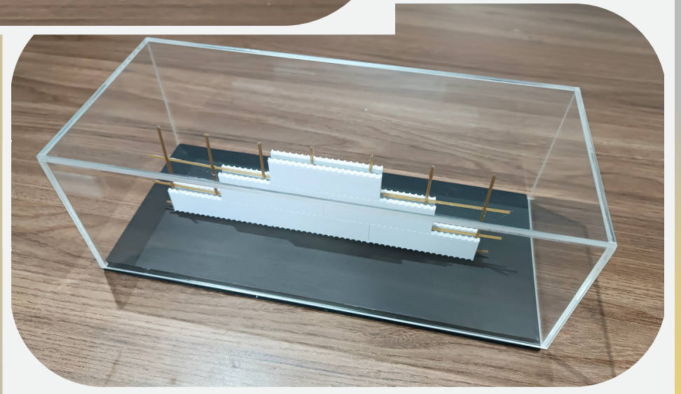
Maquete: Estrutura de um Bloco ICF (Insulating Concrete Forms)
